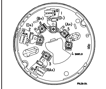
Figura 1. Distribución de los terminales
