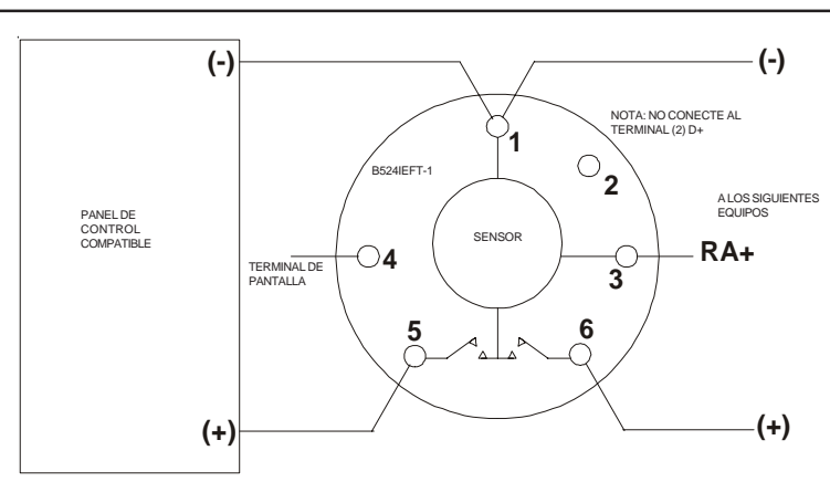
Figura 3. Diagrama de cableado típico
