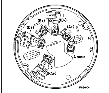
Figura 1. Schema dei terminali
